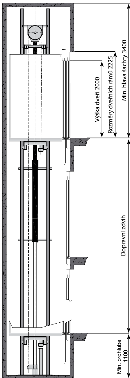
SVISLÝ ŘEZ
